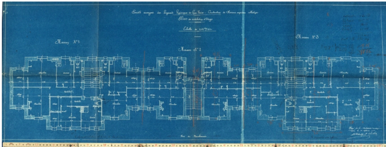
314 WP 87, 1911 permis 732, plan des étages de l'immeuble collectif rue du Bourbonnais
