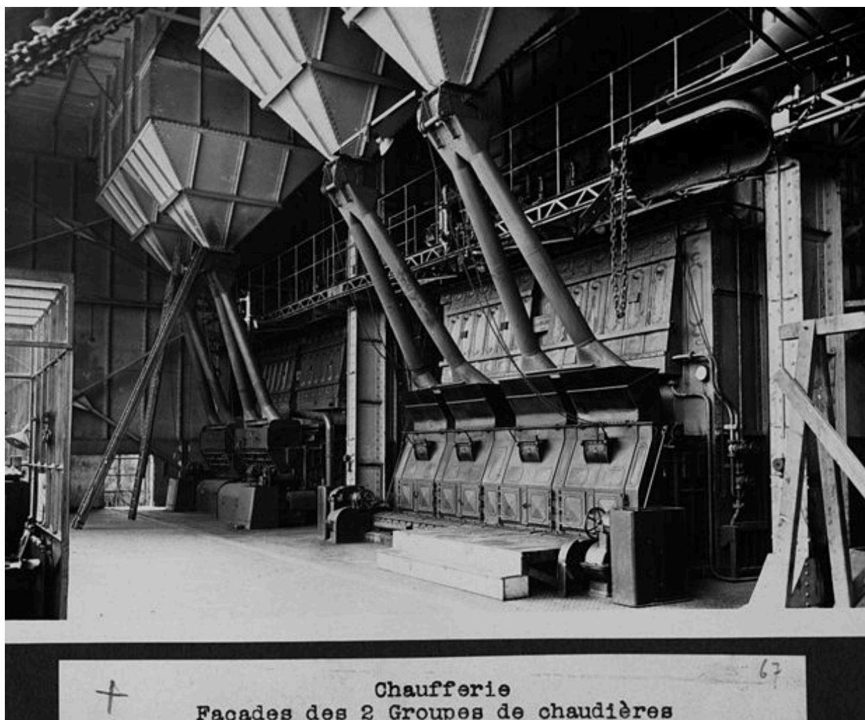
Chaufferie. Façades des deux groupes de chaudières. Photogr., vers 1960
