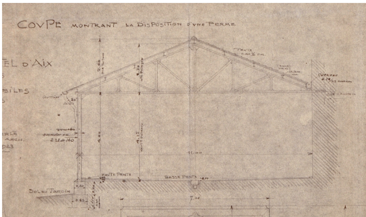
Plan, 1923. Détail sur la coupe
