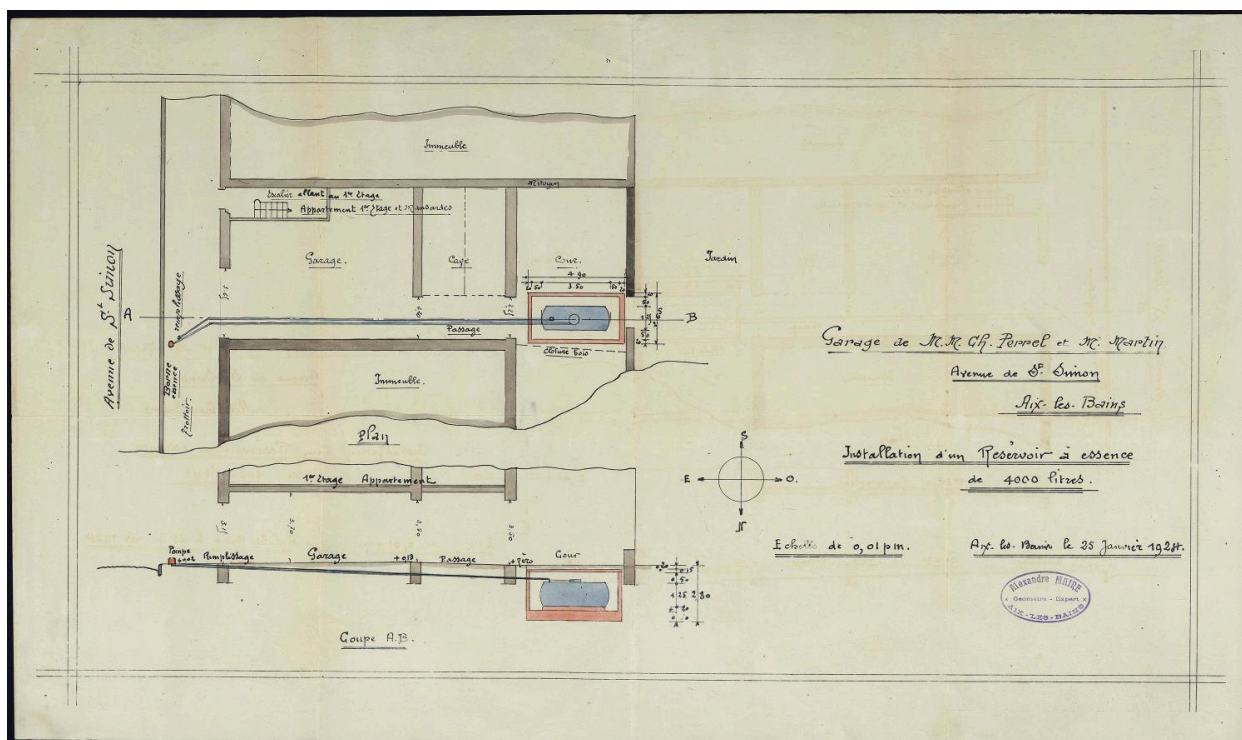
Garage Perrel et Martin, plan pour l'Installation d'un réservoir à essence
