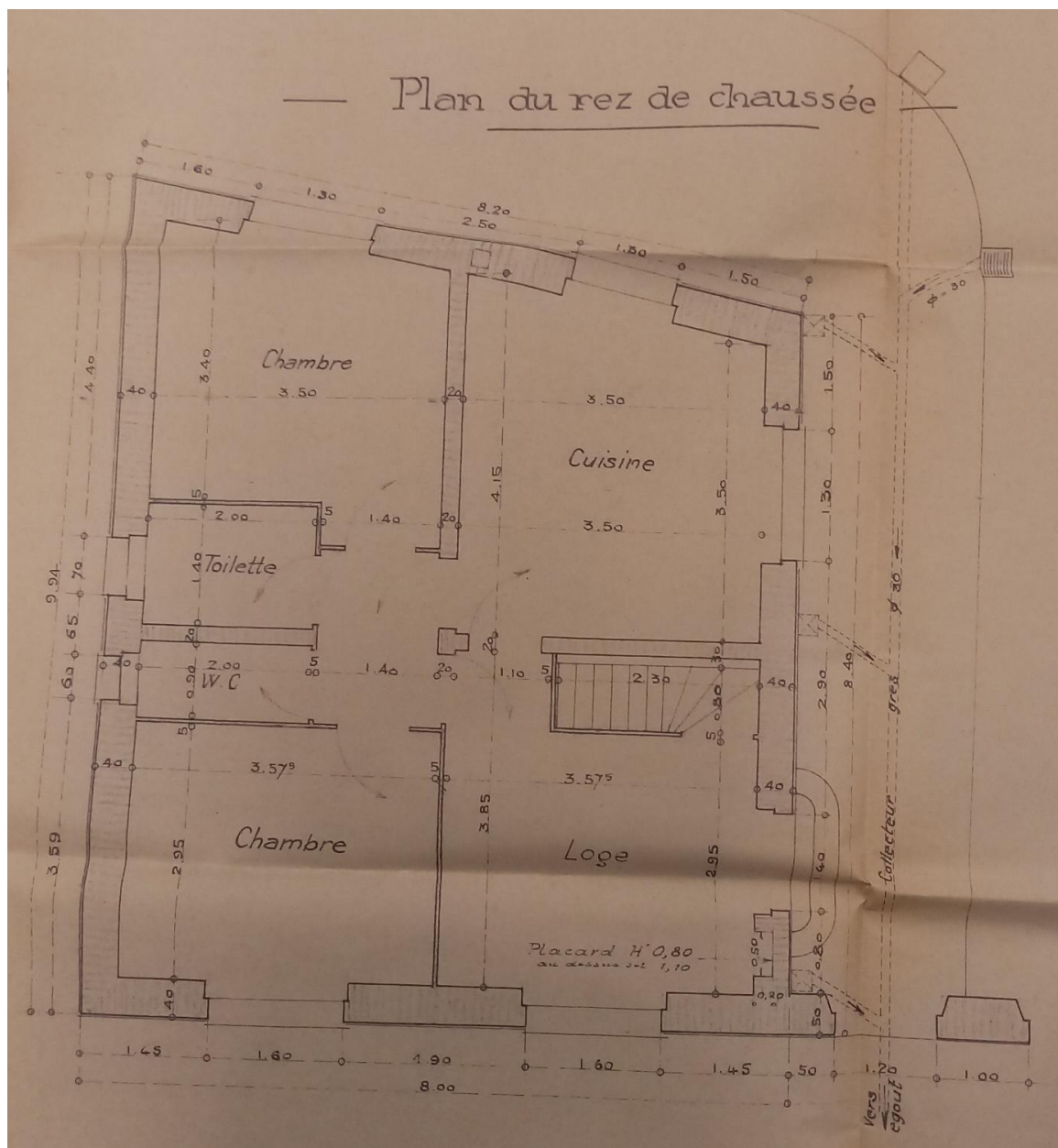
Plan du rez-de-chaussée. Maison du gardien, 1937 (détruit)
