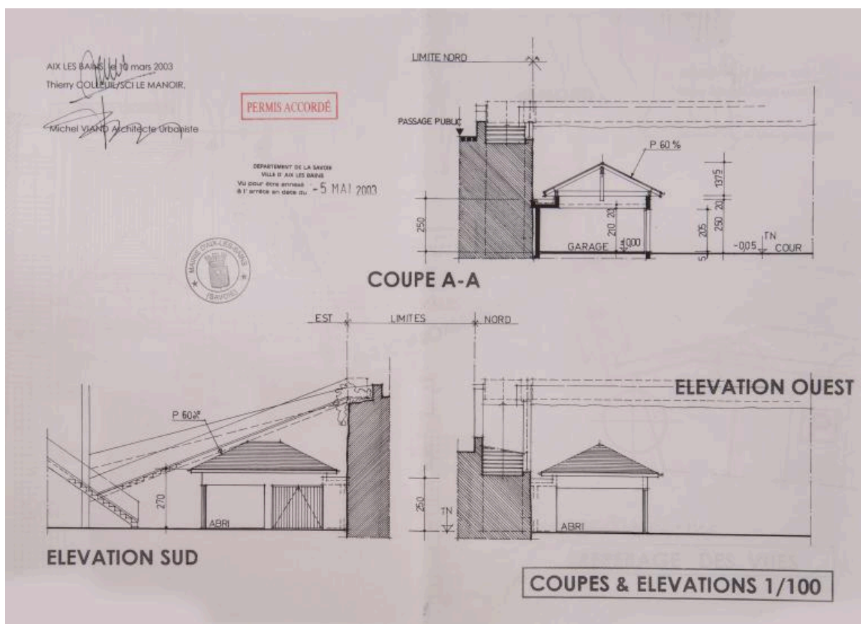
Garage, 2003 : coupe et élévations
