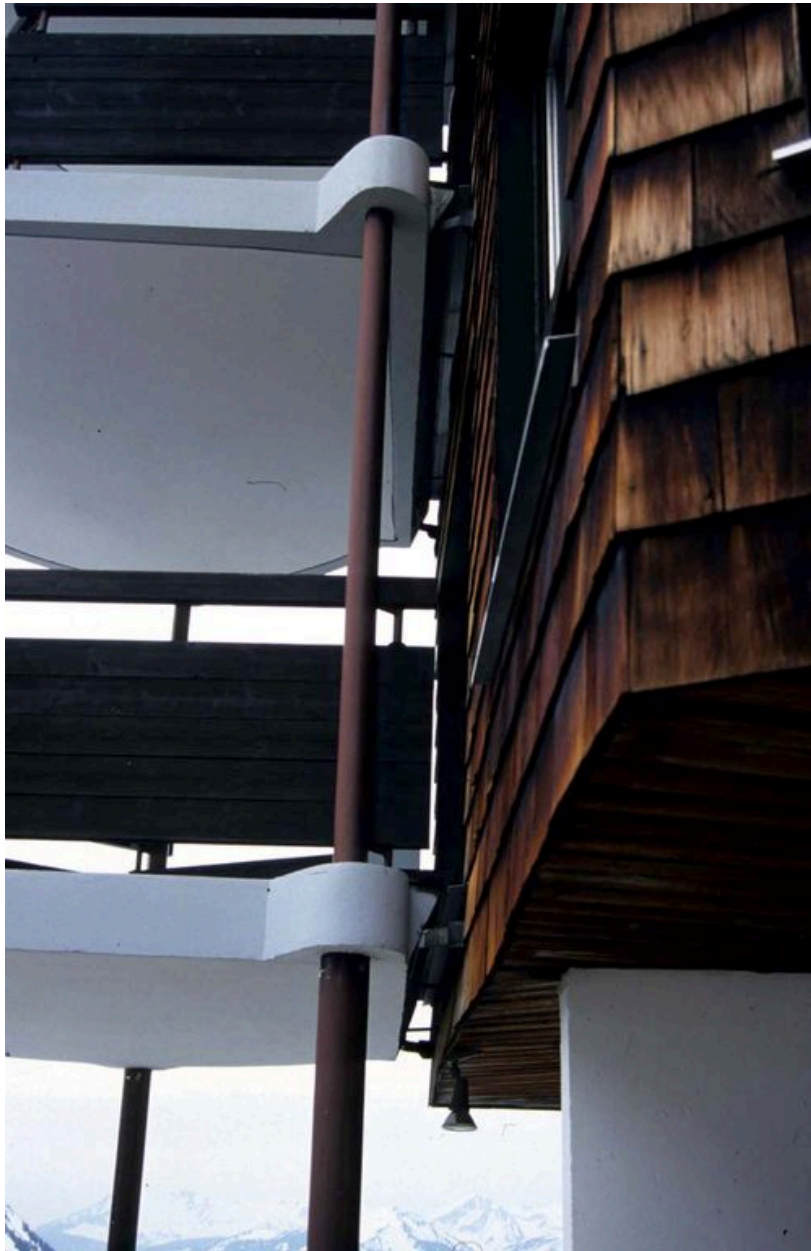
Détail des fixations des balcons
