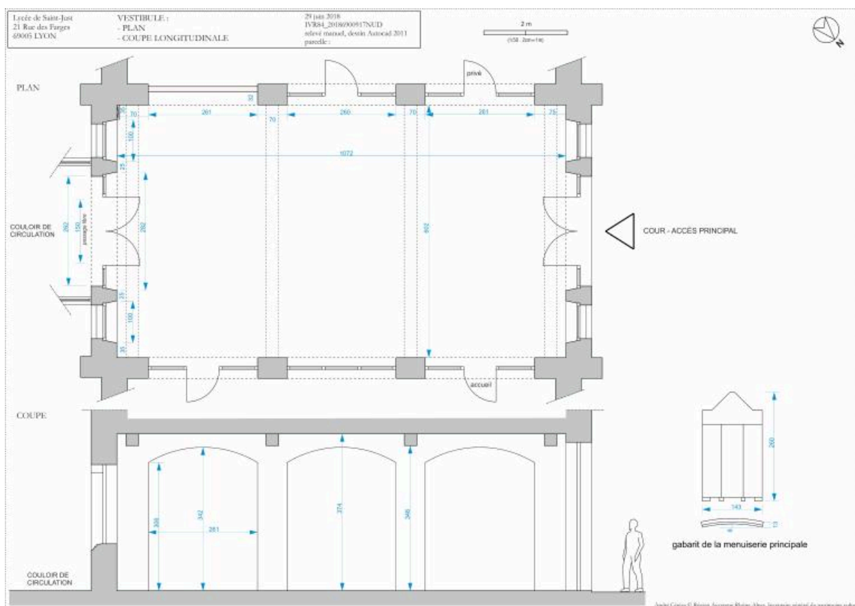
Vestibule : plan et coupe longitudinale (Dess. A. Céréza, 2018)
