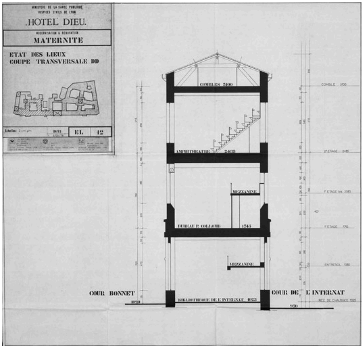
Modernisation et rénovation, maternité. Etat des lieux. Mortamet/Vidal/Manhes. SLETTI. BETSE Caillaud. Coupe transversale DD, 6 mars 1978
