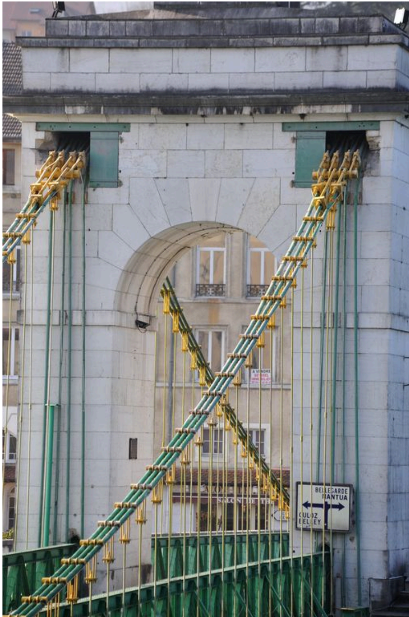
Pile centrale, vue partielle : ancrage des câbles porteurs sur l'arc monumental (depuis la rive gauche)
