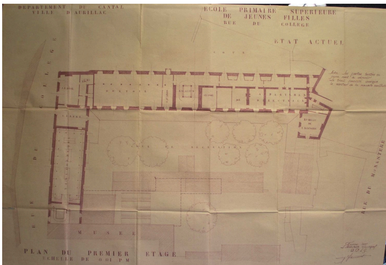
Plan du 1er étage : état des lieux, J. Brunot, 1937 (AD Cantal, 2 O 14/13-5)
