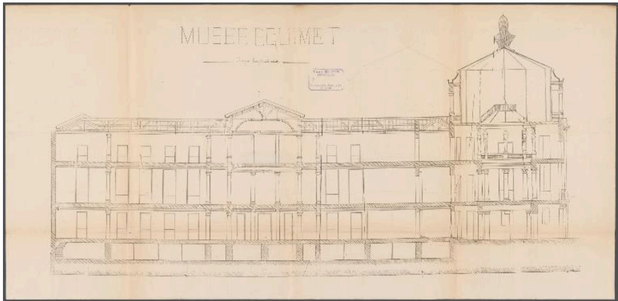
Coupe longitudinale, Tony Blein architecte, 19 mars 1912. Les caryatides de la rotonde sont encore en place. AC Lyon, 515 WP 6 2
