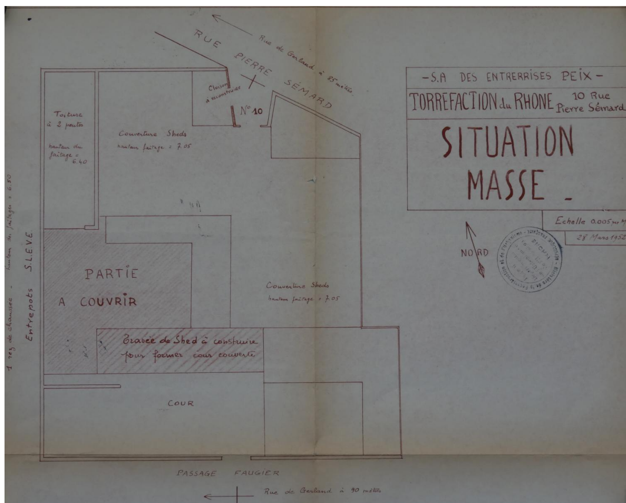
Plan masse de la société Torréfaction du Rhône, 1952 (ACL : 345W1048)
