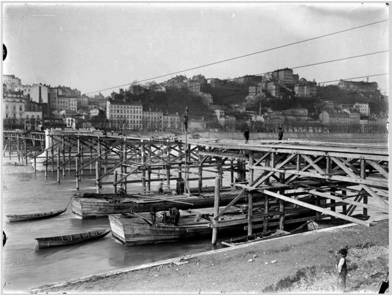
La construction du pont de la Boucle. Les premières structures du tablier. [1902]. 1 photogr. : n. et b. (AM Lyon. 15 Ph 1805)
