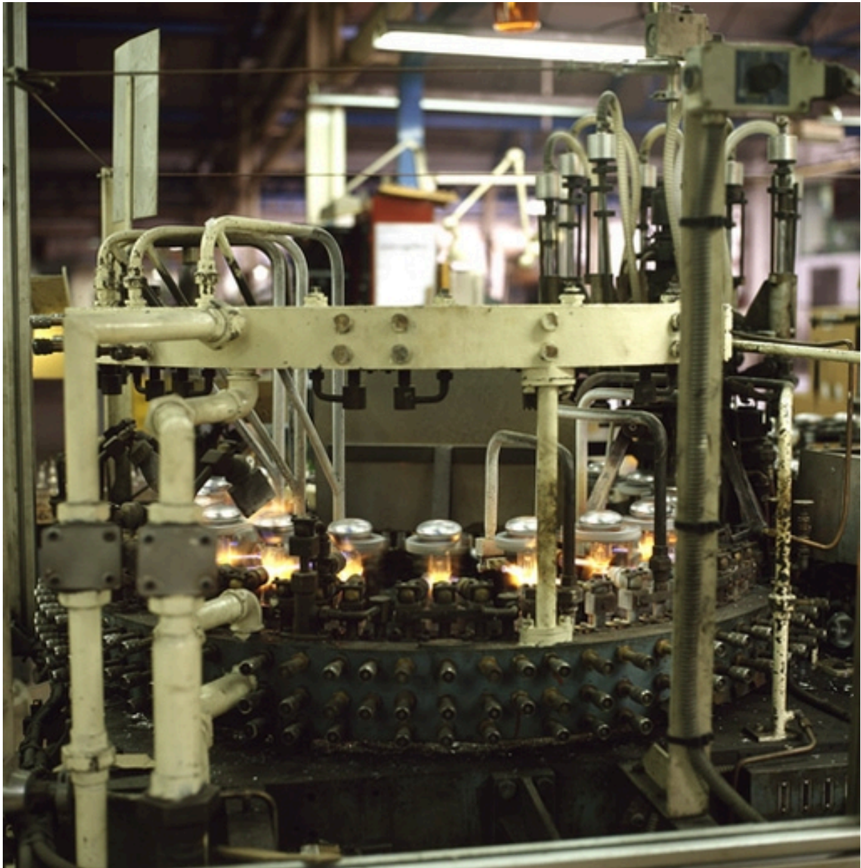
Détail machine
