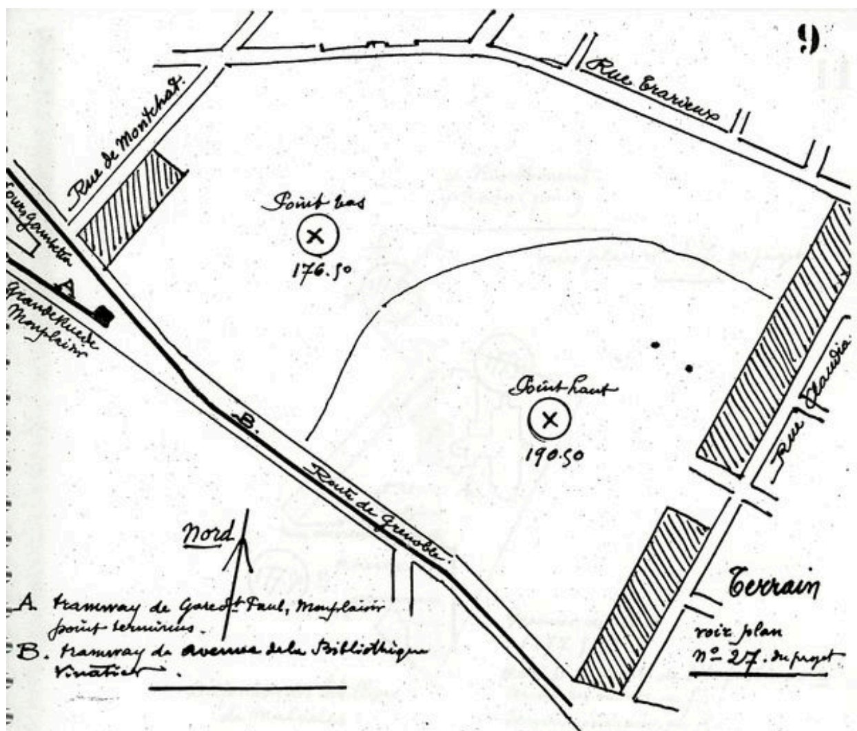
Topographie du site de Grange-Blanche / Tony Garnier, 1910
