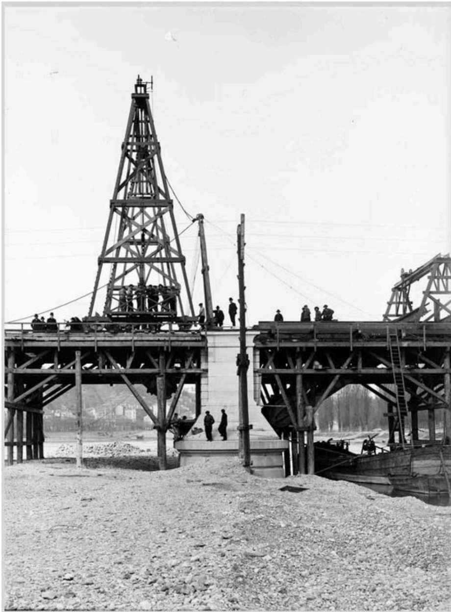
La construction du pont de la Boucle. La pile reposant sur l'îlot central du Rhône. [1903]. 1 photogr. : n. et b. (AM Lyon. 15 Ph 1815)
