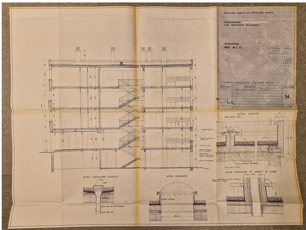
Coupe des bâtiments B et C de la rue Bernard-Brunhes et détails, par Daniel Michelin, 1967.
