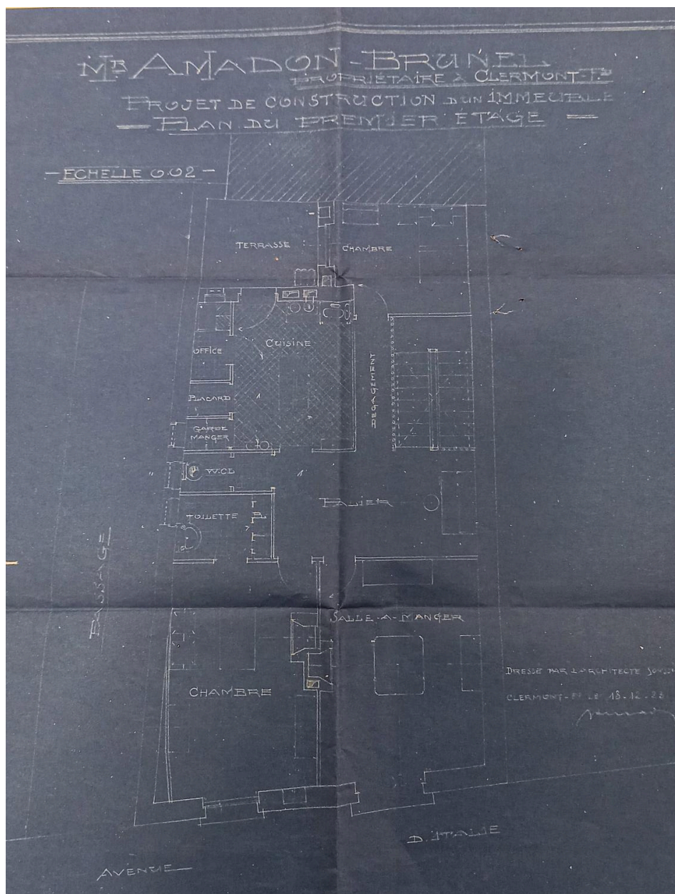
Plan du premier étage, 19 avenue d'Italie
