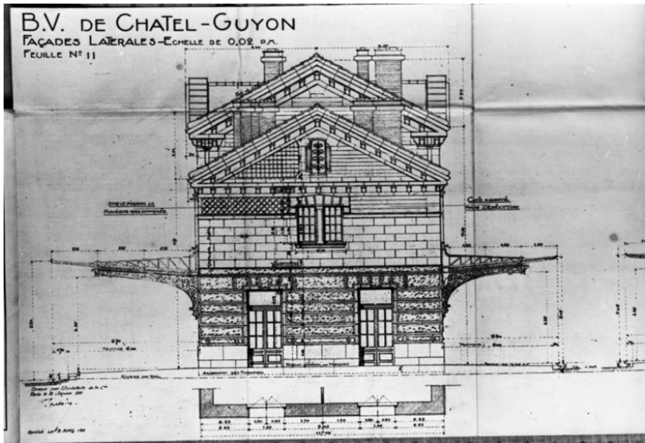
Gare de Châtel-Guyon. Bâtiment des voyageurs. Façades latérales.
