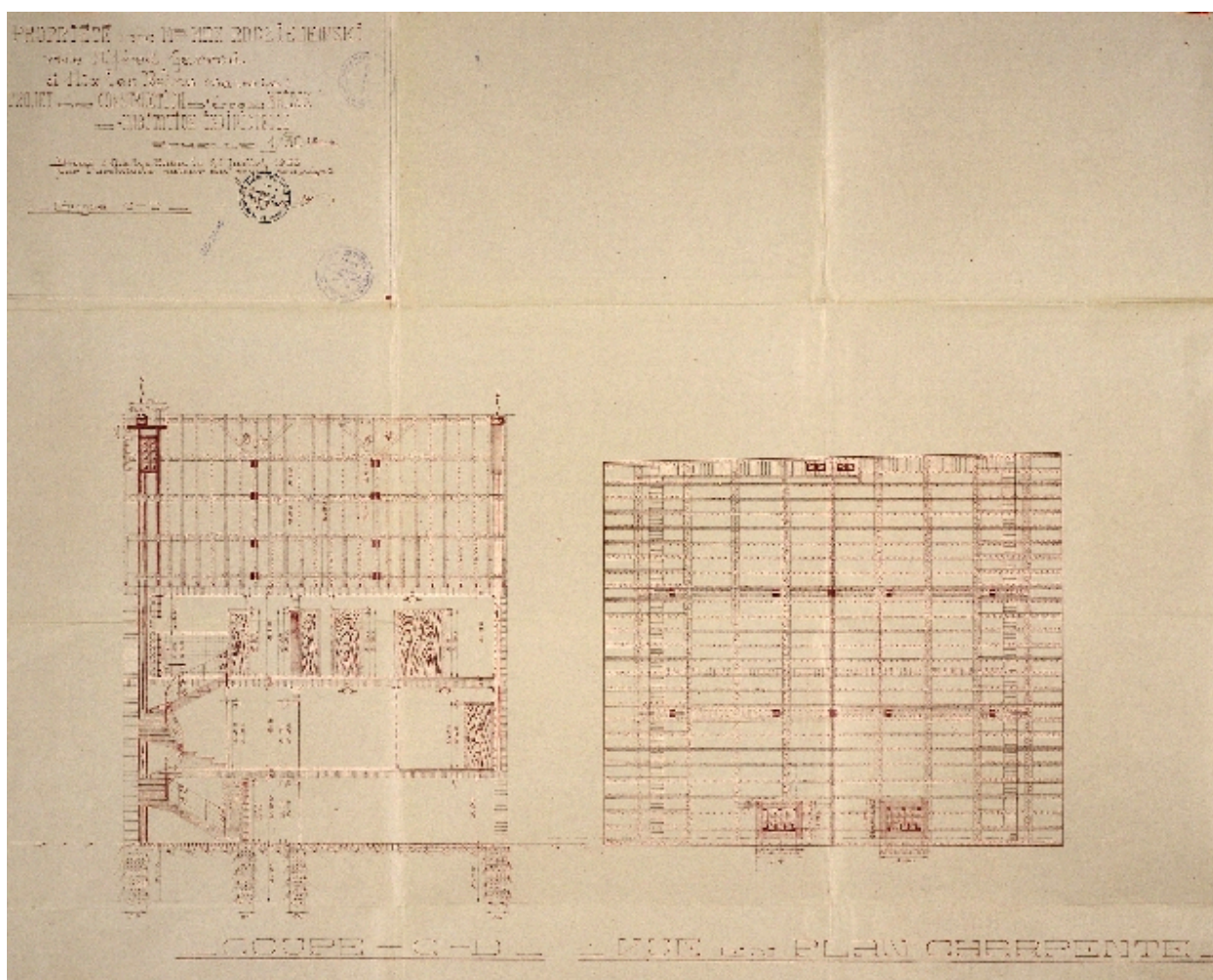
Coupe et plan des charpentes
