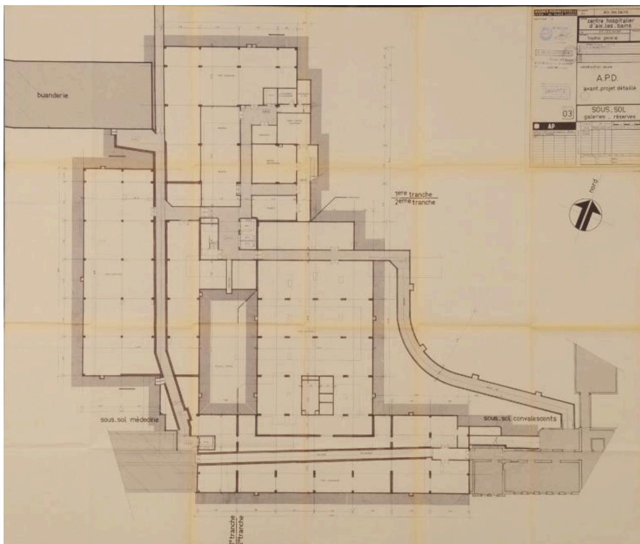
Plan des sous-sols
