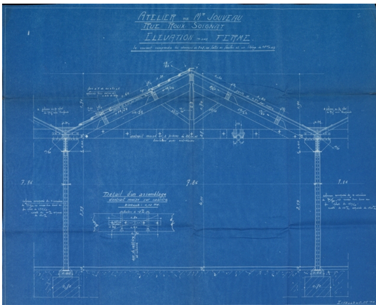
AC Lyon : 344 WP 083 PCA n°0249, détail d'une ferme du hangar de M. Jouveau par M. Pinet, 1920
