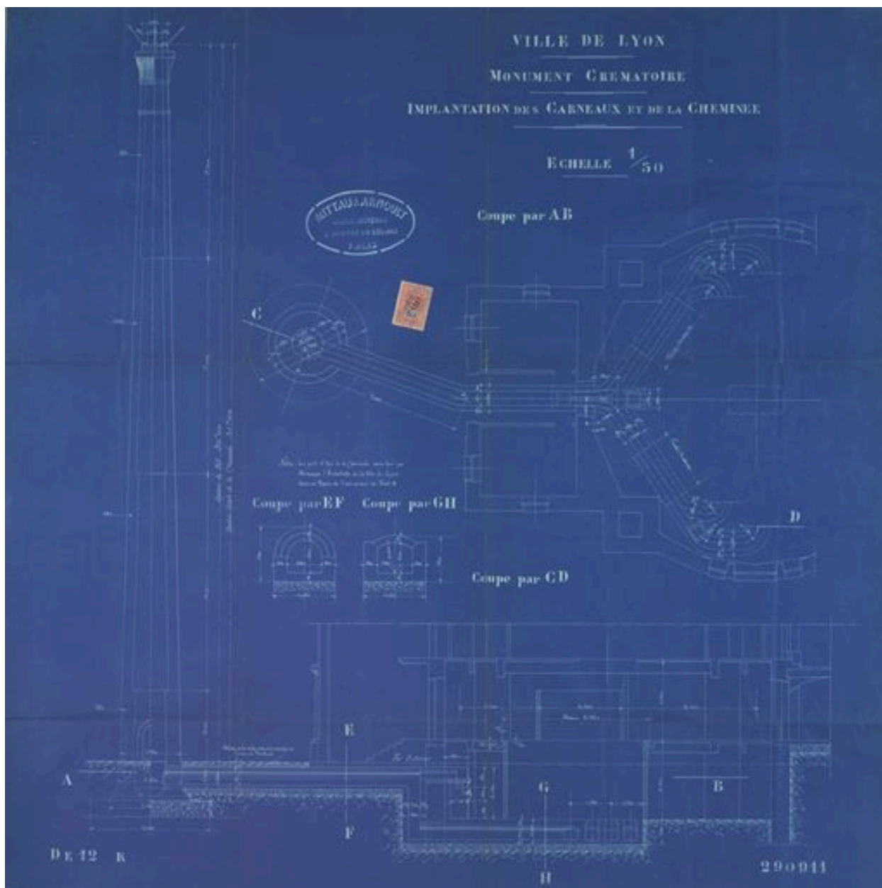
Implantation des carneaux et de la cheminée
