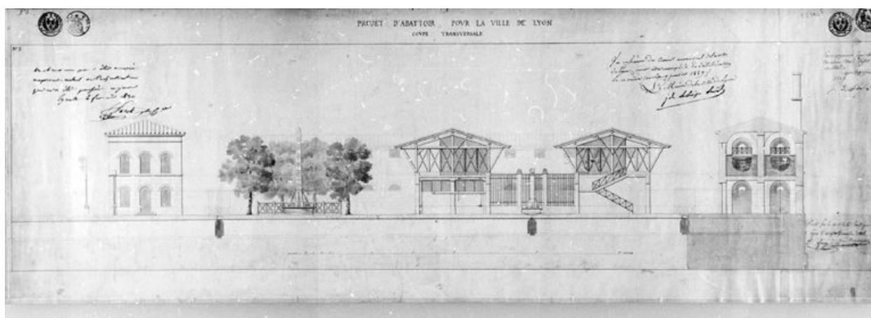
Projet d'abattoir. Coupe transversale / L. Dupasquier et V. Farge, 20 novembre 1828 (AC Lyon. 1 S 184/1)
