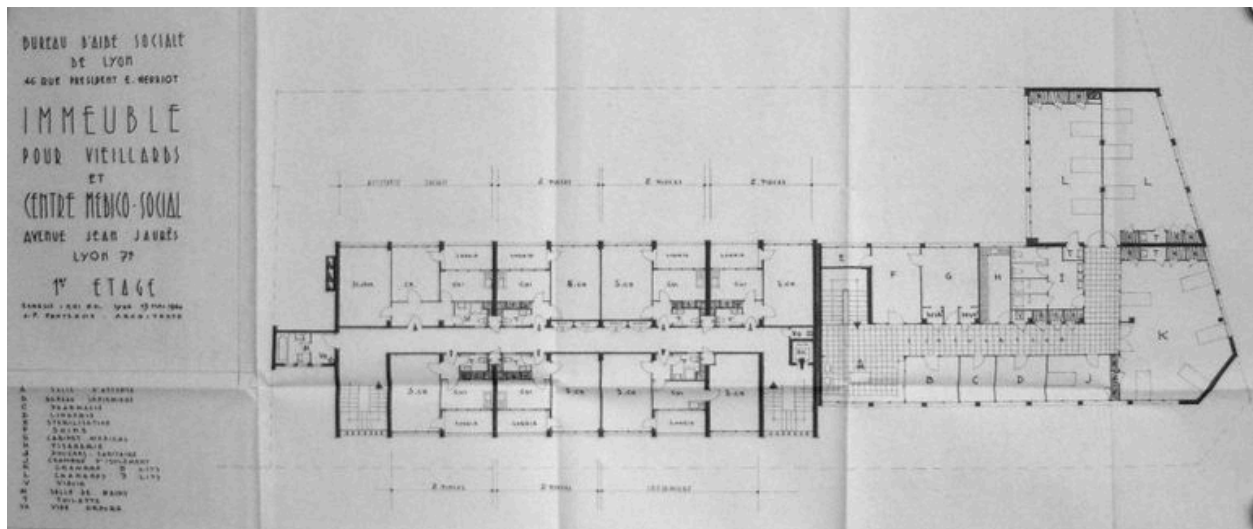
Plan des étages, immeuble pour vieillards et centre médico-social, 13 mai 1960 par J.P. Fonterme architecte, échelle 1/100. (Arch. mun. Lyon)
