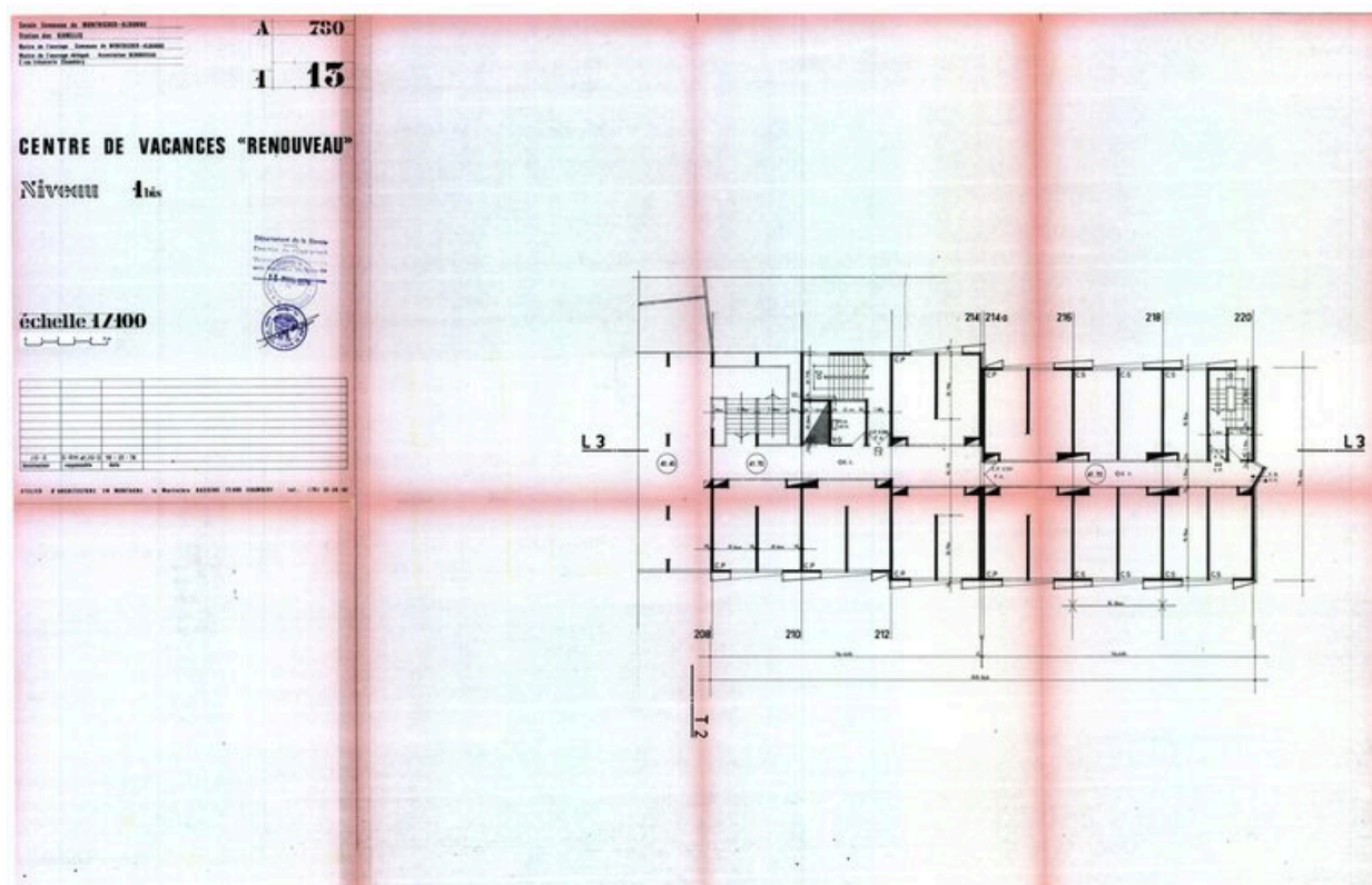
Plan du niveau 1bis (bâtiment C) / Atelier d'Architecture en Montagne, Guy Rey-Millet, Jean-Gustave Orth, 18 janvier 1973 (AC Montricher-Albanne)
