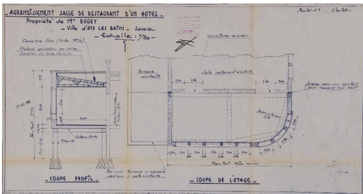
Agrandissement salle de restaurant : coupes, 1966
