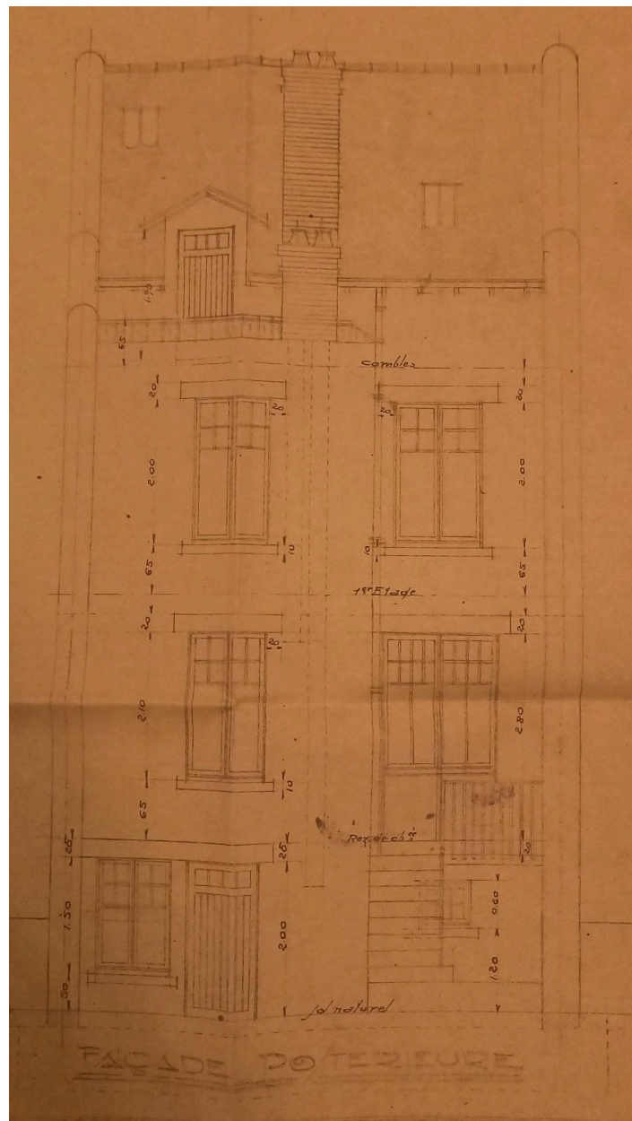
Elévation postérieure du 23 boulevard Cote-Blatin
