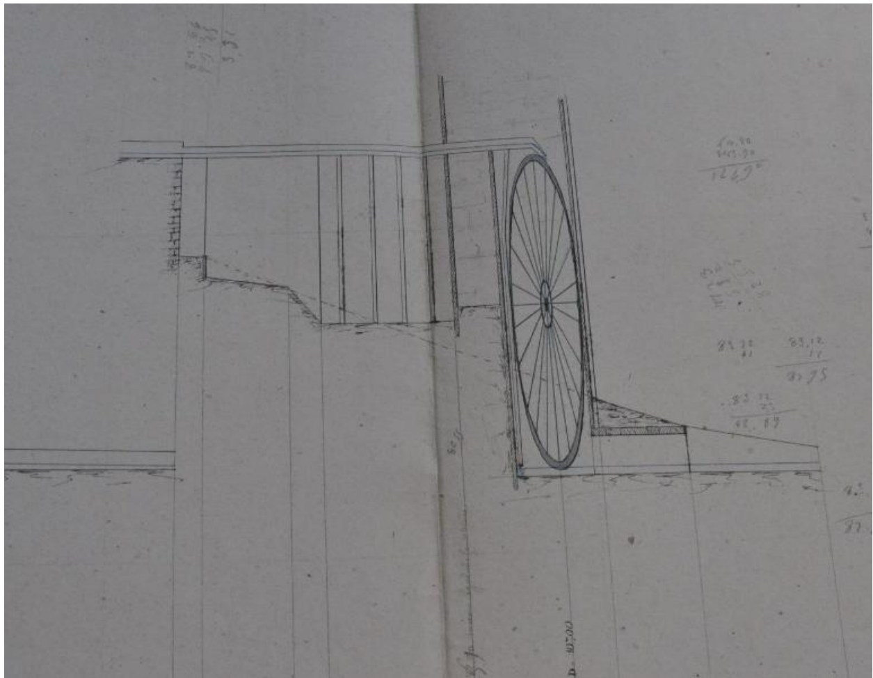
Plan des roues du moulin Jallabert, 1864 (FR.AD073, 49SPC1).
