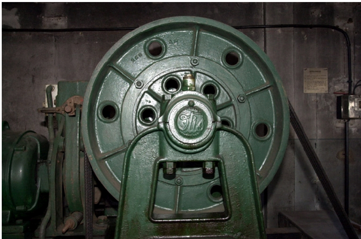
Détail alimentation monte-charge
