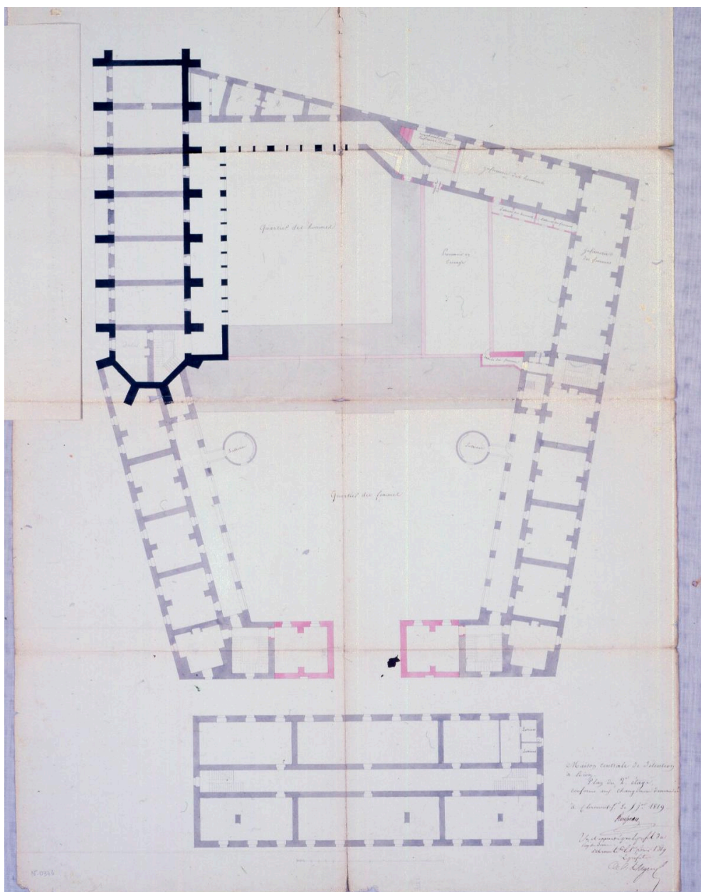
Maison centrale de détention à Riom. Plan du deuxième étage, lavis rose et violet, encre noire, sans échelle, 1819, par Rousseau.
