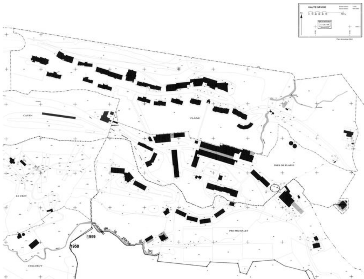
Plan de situation de la station inférieure de la télécabine des Grands Vans. Extrait du plan cadastral d'Arâches-la-Frasse. 1 : 1000
