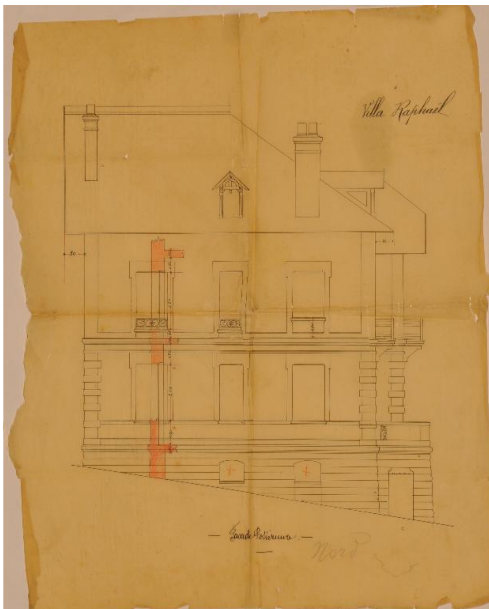
Elévation nord
