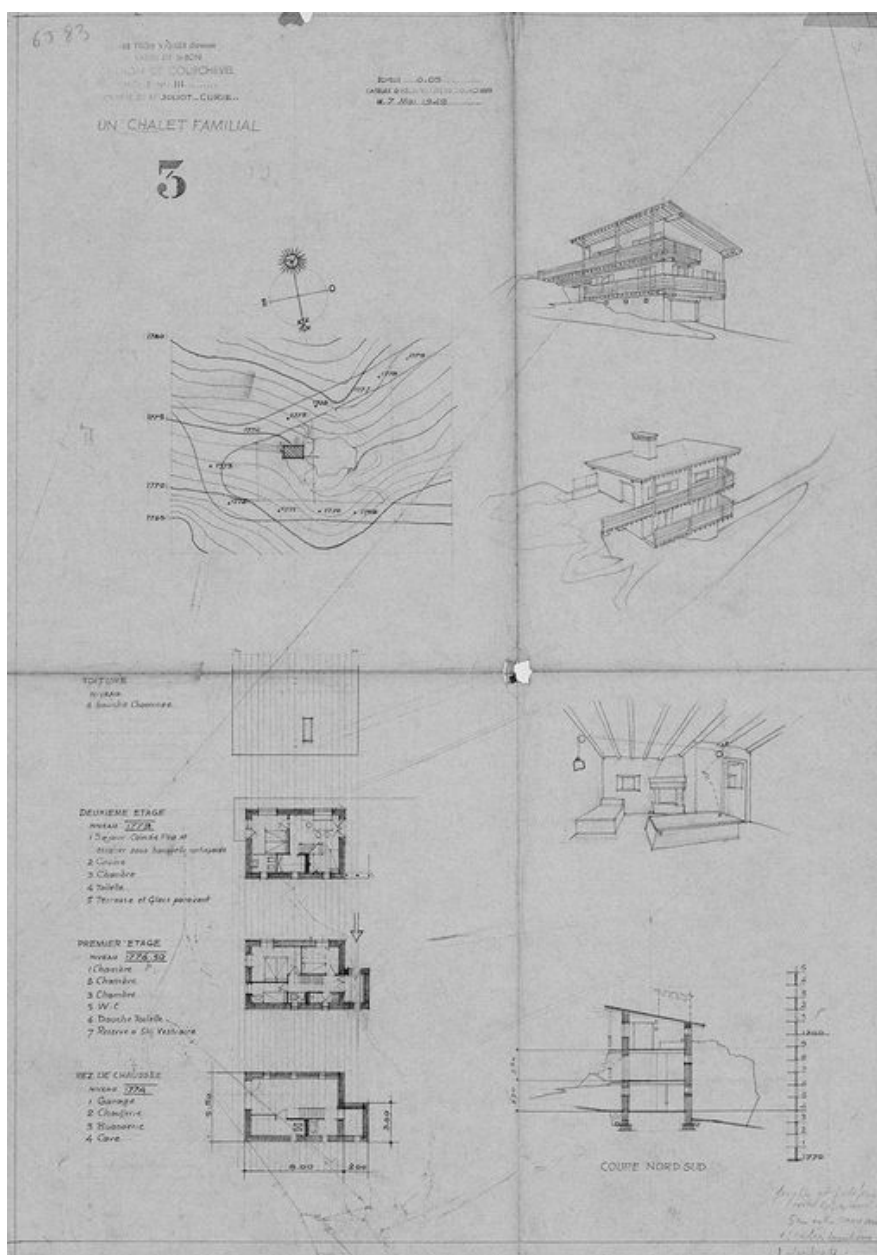
Un chalet familial. Plans, coupes, élévations. Esquisse / Atelier d'Architecture de Courchevel, 7 mai 1949 (AD Savoie. 6J 83)
