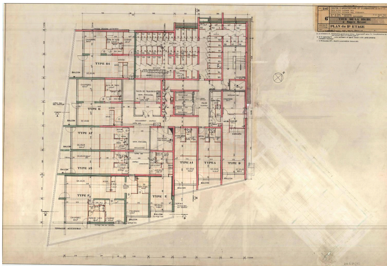
La Tour de la Biche, projet exécuté, plan du 2e étage, janvier 1970, Faye et Tournaire architectes (AD63, 217 Fi 81 / 15).
