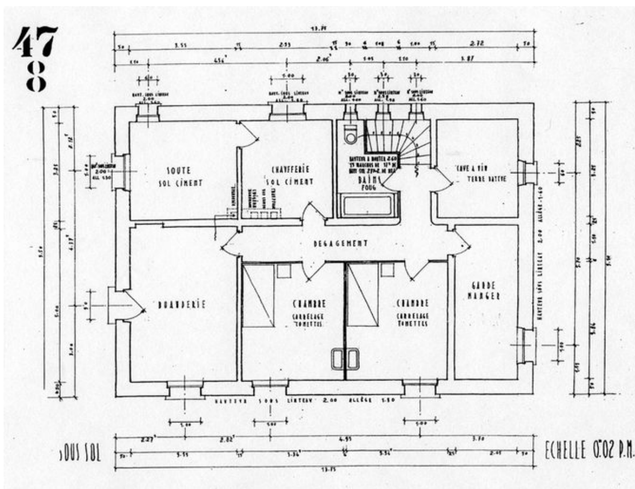
Plan du sous-sol. Henry Jacques Le Même, [1928] (Dossier agence n° 47)
