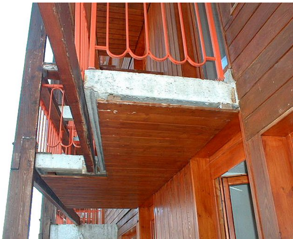
Façade ouest : les terrasses, détail de construction
