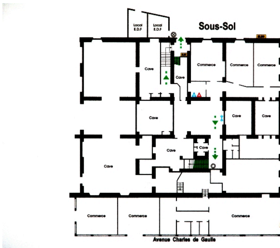
Plan du sous-sol
