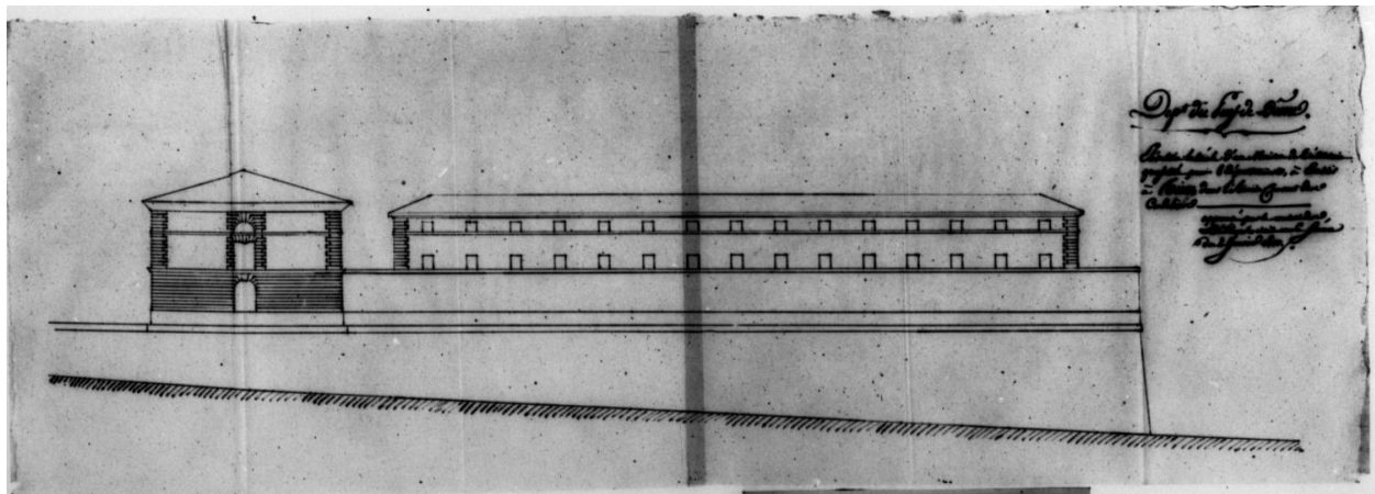
Élévation soumise au Conseil des bâtiments civils (façade nord, sur le boulevard), 1810 (AN F/21/1895).
