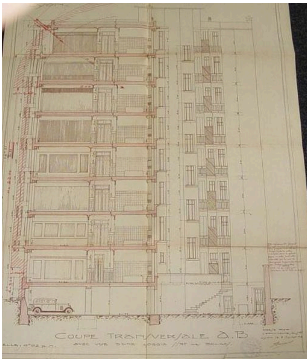
Coupe transversale / Bornarel, 1928
