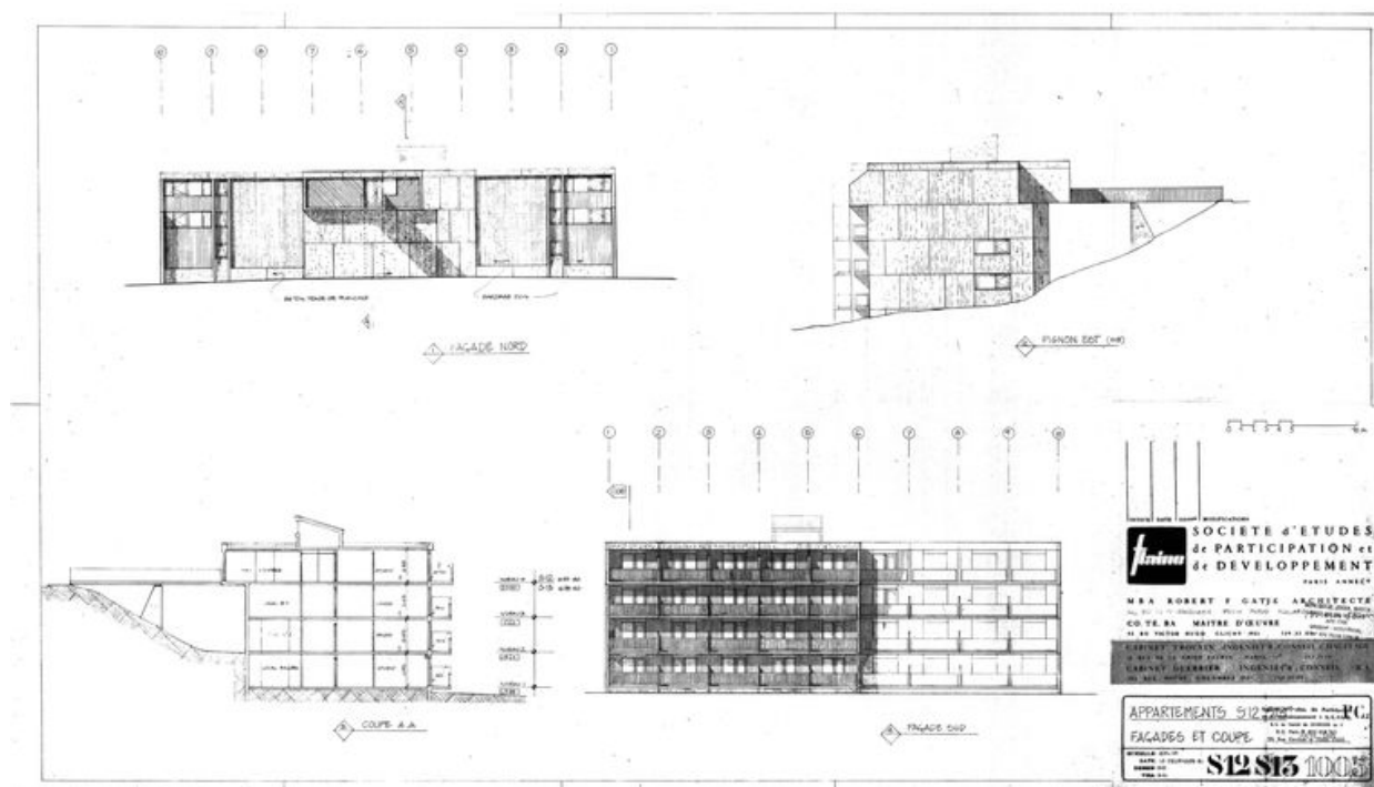
Elévations et coupe. M.B.A. Robert F. Gatje, 10 décembre 1981 (AC Arâches-la-Frasse)
