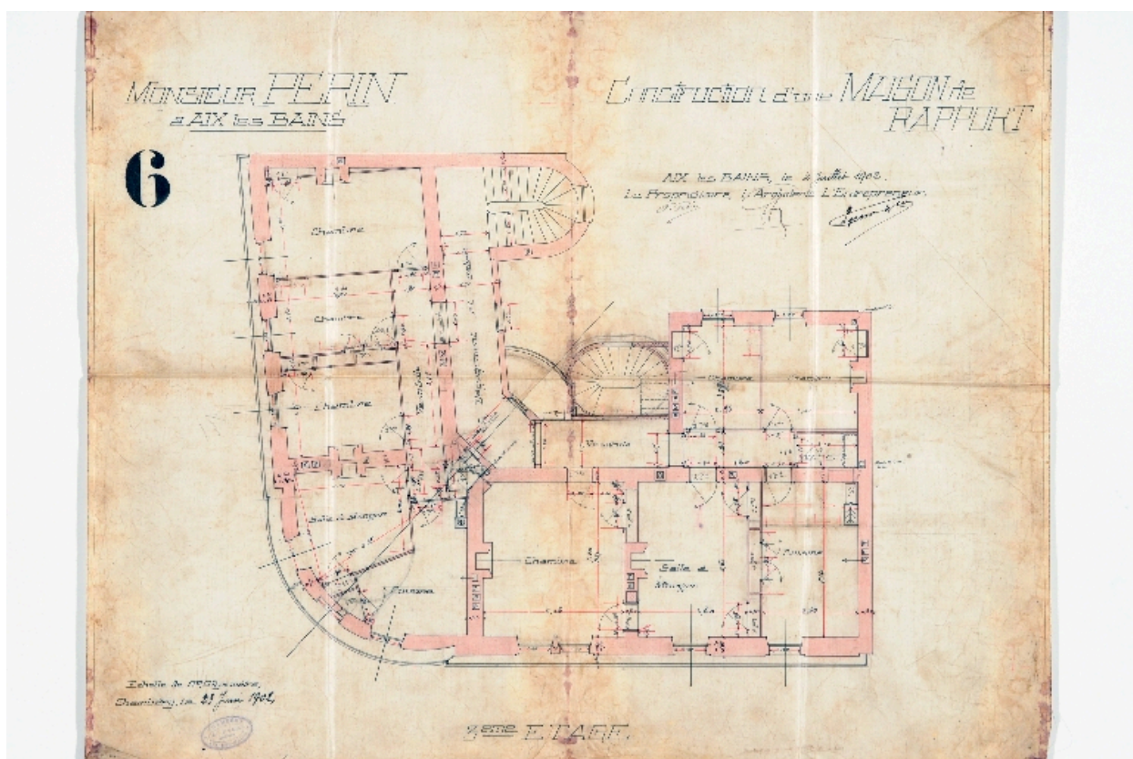
Plan du 3e étage
