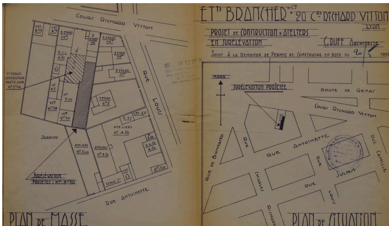
Projet construction atelier en surélévation, 1953 (ACL 348W/14)
