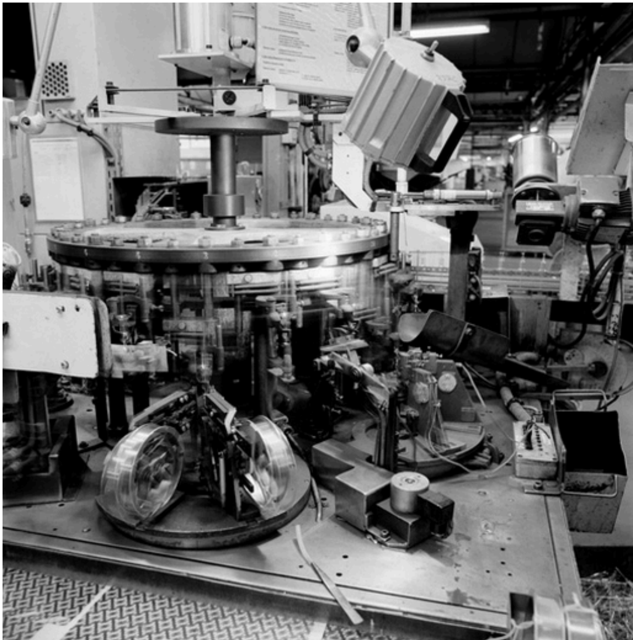
Ligne filament
