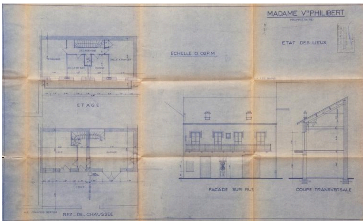
Plans, élévation et coupe, 1961
