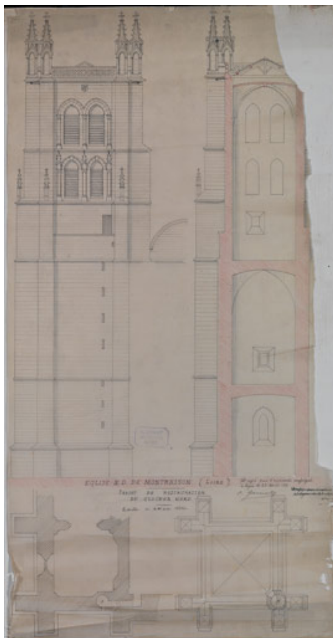
Eglise N. D. de Montbrison. (Loire). Projet de restauration du clocher nord.
