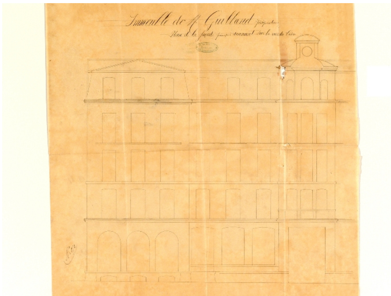
Elévation sur la rue du Casino
