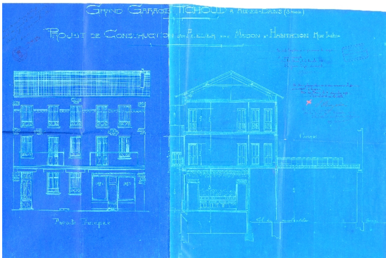
Coupe et élévation principale
