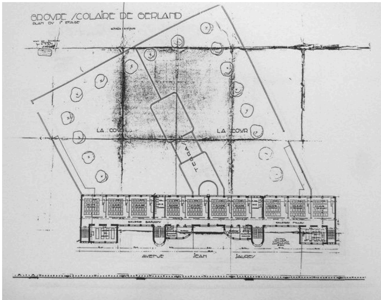
Plan du 1er étage Projet Ecole primaire de Gerland, 12 avril 1930 par V.-A. Robert et A.-E. Chollat architectes, échelle 1/100. (AC Lyon)
